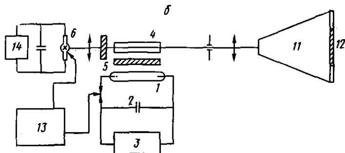
Рис. 6.1. Схема кинетической (а) и спектрографической (б) установки импульсного фотолиза. 1 — импульсная лампа; 2 — конденсатор; 3 — зарядное устройство; 4 — кювета; 5 — фильтры; 6 — спектроскопическая лампа; 7 — монохроматор; 8 — фотоумножитель; 9 — осциллограф; 10 — питание ФЭУ; 11 — спектрограф; 12 — фотоэлектронная труба; 13 — блок временной задержки; 14 — питание импульсной спектроскопической лампы
