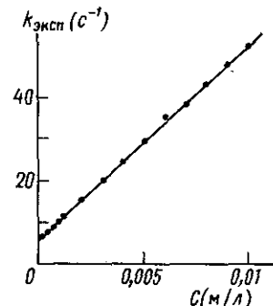
Рис. 6.23. Зависимость константы скорости превращения аниона 2,4-динитротолуола от концентрации ацетатного буфера
