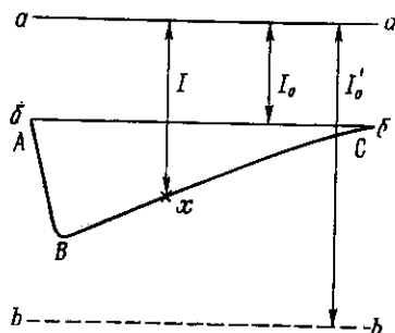
Рис. 6.15. Осциллограмма изменения поглощения исходного соединения при импульсном фотолизе
