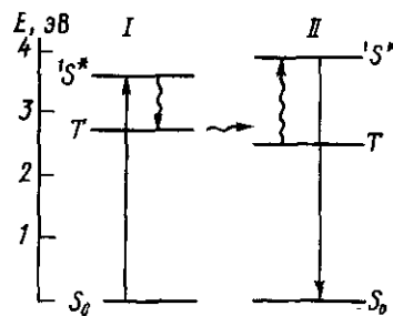
Рис. 6.5. Энергетические уровни возбужденных состояний фенантрена (I) и нафталина (II)
