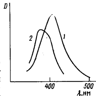
Рис. 6.13. Спектры изомерных форм о-нитротолуола, полученных при импульсном фотолизе в кислой (1) и щелочной (2) растворах
