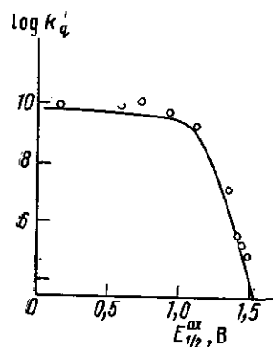
Рис. 6.9. Зависимость констант скорости тушения триплетных молекул тионина от потенциалов окисления доноров (слева направо): тетраметилпарафенилендиамина (0,16 В); п -метоксидиметиланилина (0,59 В); м -метоксидиметиланилина (0,75 В); трифениламина (0,92 В); 1,2,4-триметоксibenзола (1,12 В); 1,4-диметоксibenзола (1,34 В); 1,2,3-триметилбензола (1,42 В); 1,2-диметоксibenзола (1,45 В); 1,3,5-триметоксibenзола (1,49 В)
